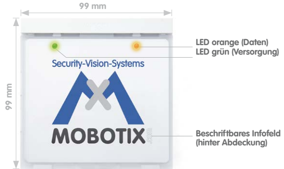
Ansicht mit entferntem Gehäusedeckel
