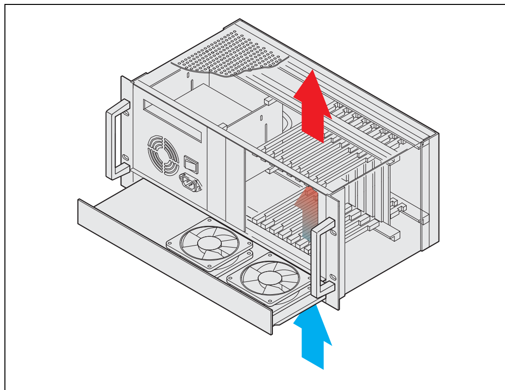
Figure 2: Entwärmung
