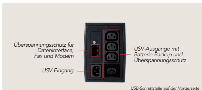
Protect alpha 450/600/800 – Rückansicht
