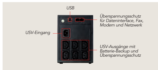
Protect alpha 1200 – Rückansicht
